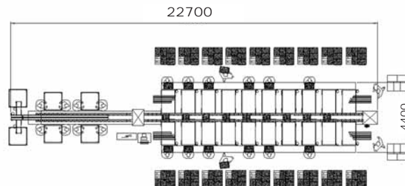
F2] Dos canales con alimentación manual Deux ligne avec alimentation manuel
