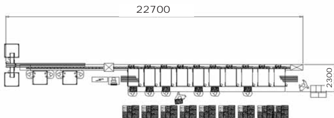
F1] Monocanal con alimentación manual Mono - ligne avec alimentation manuel
